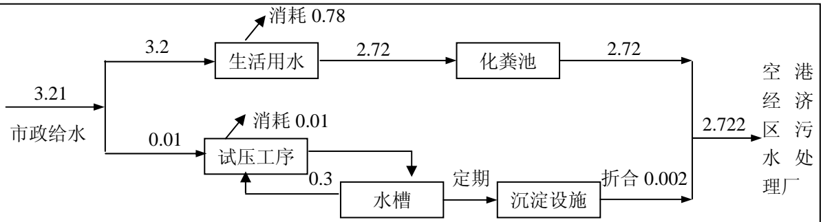
图1 本项目水平衡图（单位： \text{m}^3/\text{d} ）
